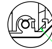
C : フレーム拡大図 / Frame cross-section
